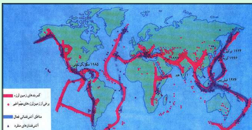
۳۸ - انځور په نړۍ کې د زلزلې او اور غورځونکي کمربند ښيي
