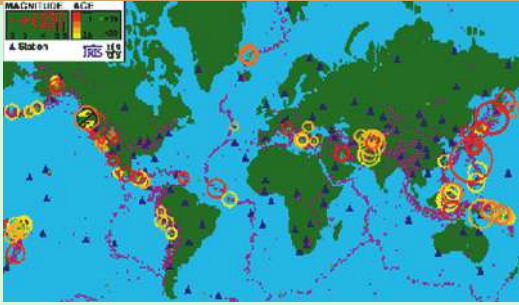
۲۷ - انځور د زلزلو مرکز ښيي
