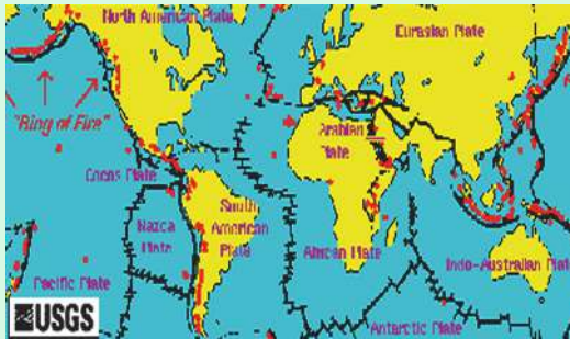
۲۸ - انځور تکتونیکي هستې ښيي
