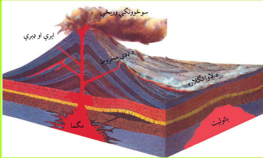
۳۷- انځور اور غورځوونکي ښيي
