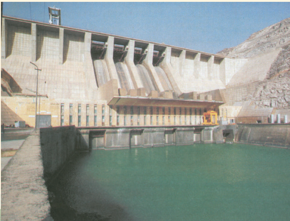
فابریکه تولید برق آبی نغلو
